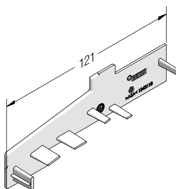
Торцевые колпачки для профиля подставочного 121
