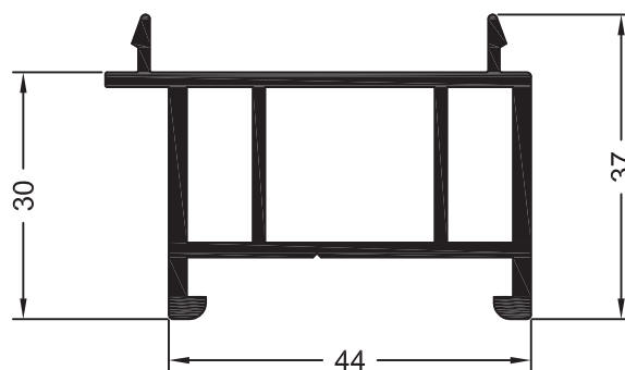
Профиль подставочный 33
