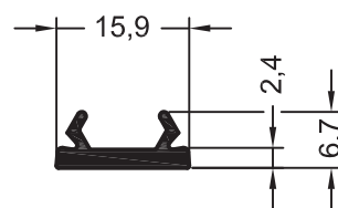
Заглушка паза прибора запираания 16
