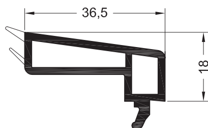
Штапик 36,5
