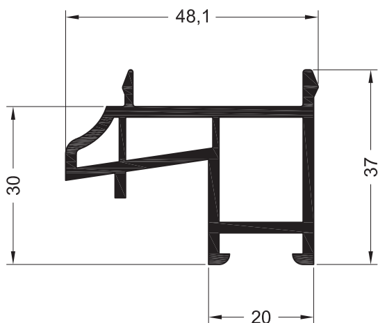
Профиль подставочный 42
