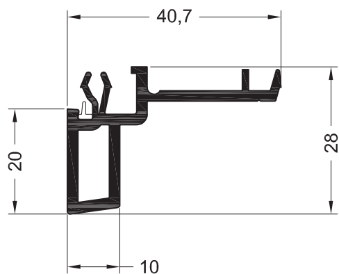
Профиль подставочный 20/10
