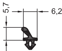
Уплотнение притвора ремонтное 1865280 @ 1865600 @ 400 EPDM
