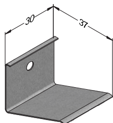
Скоба 1/70 Сталь пружинная
