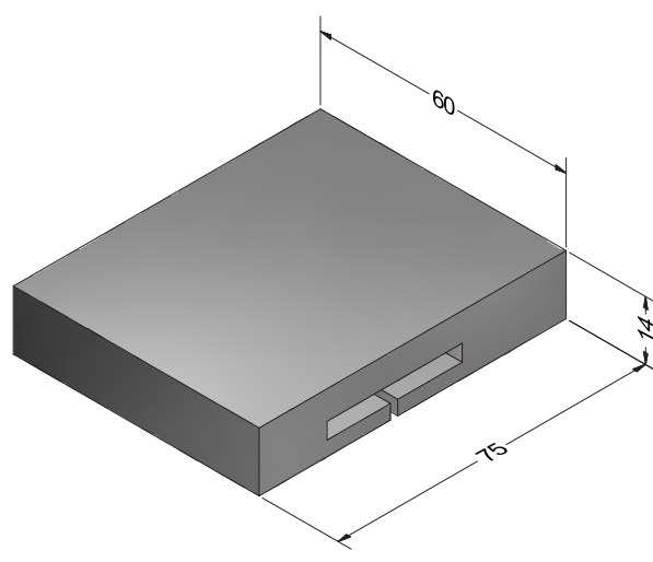
Уплотняющая вставка профиля компенсирующего 2 EPDM вспененный
