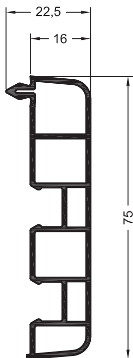
Наличник 75
