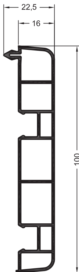
Наличник 100
