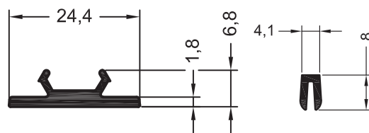
Заглушка паза прибора запираания 24
