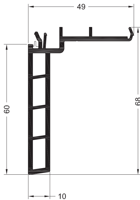
Профиль подставочный 60/10
