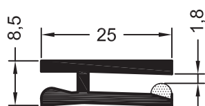
Профиль для крепления компактной плиты
