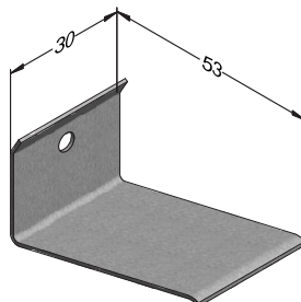
Скоба 1/86 Сталь пружинная
