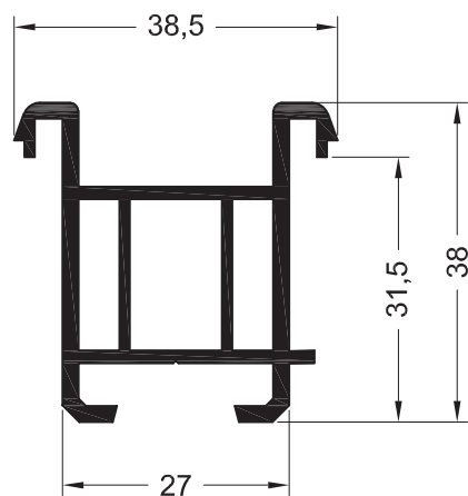
Профиль подставочный 30
