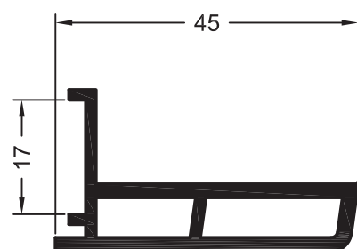
Нащельник 45
