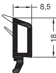
Штапик 8,5
