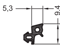
Уплотнение для стекла № 66 1835151 200 SIK
