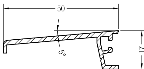
Планка порога с козырьком и пазом для уплотнения
