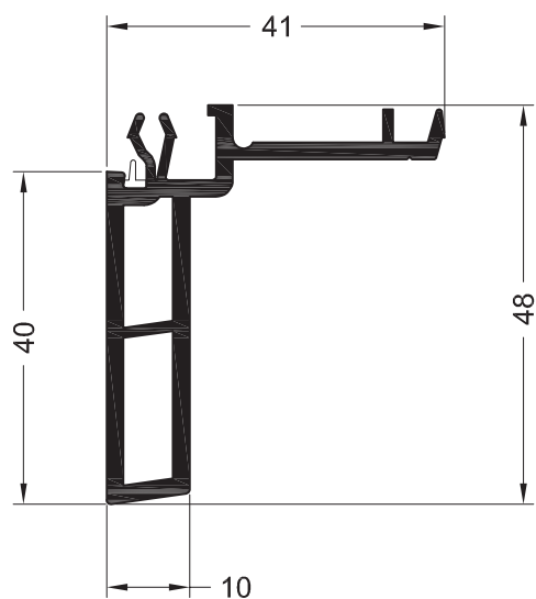
Профиль подставочный 40/10
