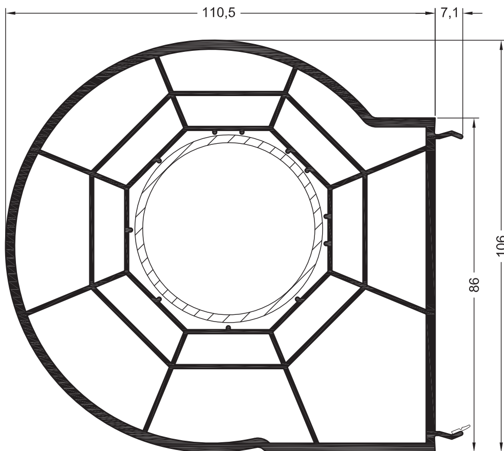
Профили для эркерных окон
