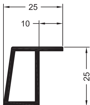
Нащельник 25
