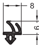
Уплотнение притвора 1835171 200 SIK
