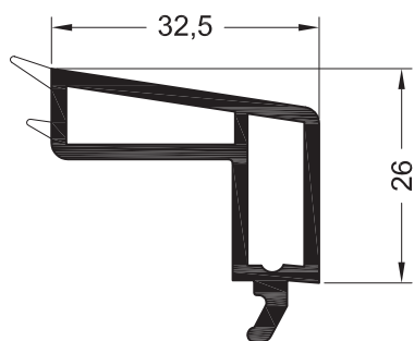
Штапик 32,5 для глухого остекления
