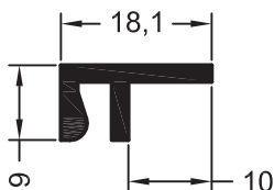
Профиль ограничитель
