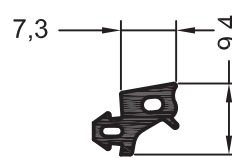
Уплотнение для стекла № 68 1835161 @ 150 SIK
