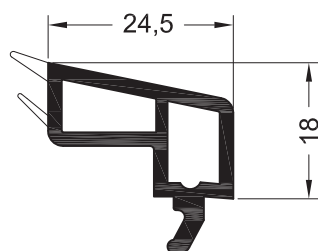
Штапик 24,5
