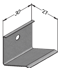
Скоба 1/60 Сталь пружинная
