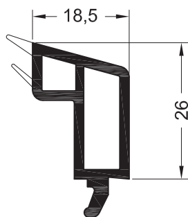
Штапик 18,5 для глухого остекления
