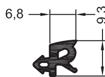
Уплотнение для стекла № 67 1865012 @ 1865560 @ 300 EPDM
