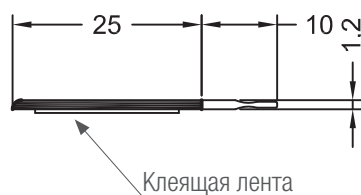
Наличник (для помещений)
