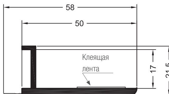
Нащельник 50
