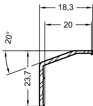
Защитная планка порога 1/86
