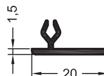
Профиль силиконового шва 2
