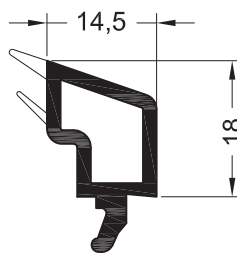
Штапик 14,5
