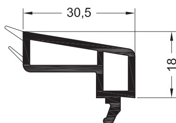
Штапик 30,5
