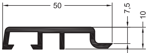
Нащельник 50
