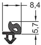
Уплотнение притвора 1884952 400 EPDM 1865535 400 EPDM
