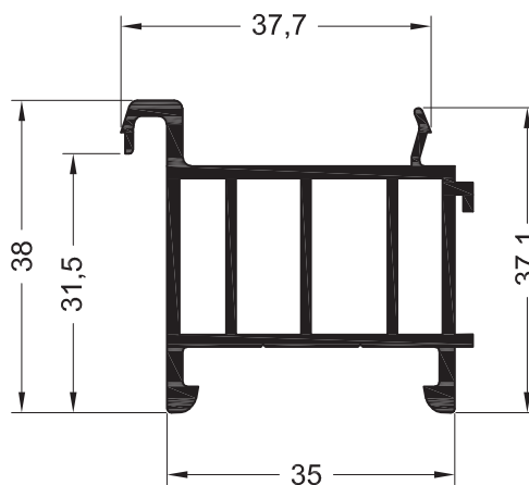
Профиль подставочный 35
