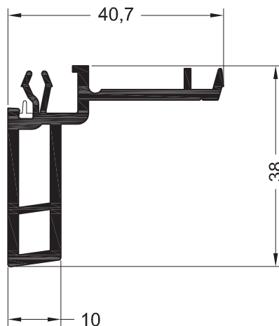
Профиль подставочный 30/10
