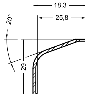
Защитная планка коробки 76/80 BriD
