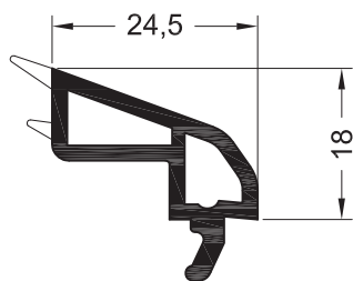
Штапик фигурный 24,5
