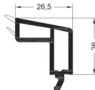
Штапик 26,5 для глухого остекления
