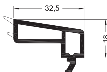
Штапик 32,5
