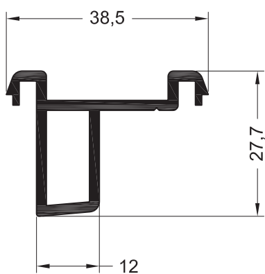
Профиль подставочный ремонтный
