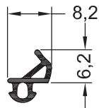
Уплотнение притвора 1330101 1003 500 EPDM 1330101 1004 500 EPDM
