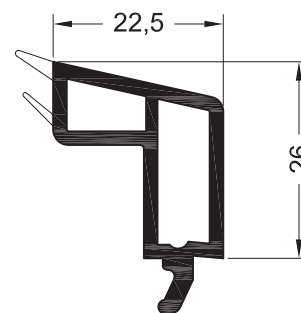
Штапик 22,5 для глухого остекления
