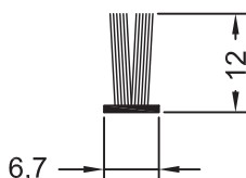
Уплотнение щеточное 6,7 x 12 (для направляющей жалюзи 533180)
