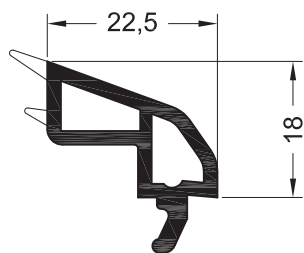
Штапик фигурный 22,5
