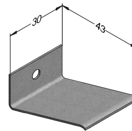
Скоба универсальная Сталь пружинная
