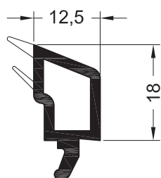
Штапик 12,5
