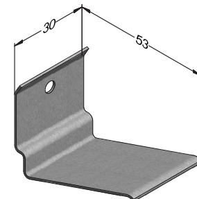
Скоба 2/86 Сталь пружинная
