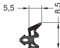
Уплотнение для стекла ремонтное 1865290 @ 1865610 @ 200 EPDM
