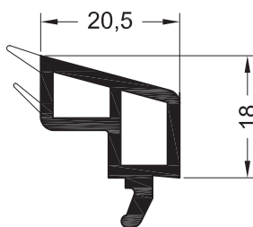
Штапик 20,5
