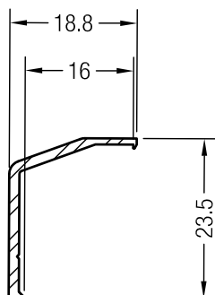
Защитная планка порога 1/70
