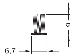
Уплотнение щеточное 6,7 x 9 (для слезника 21, 351558)
