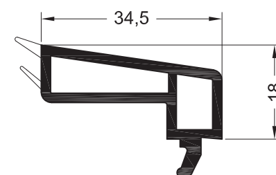
Штапик 34,5
