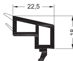
Штапик 22,5
