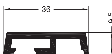
Внутренний нащельник на стык в окне со штапелом
