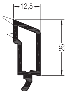
Штапик 12,5 для глухого остекления
