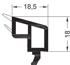
Штапик 18,5
