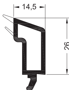
Штапик 14,5 для глухого остекления
