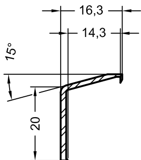
Защитная планка порога 1/60
