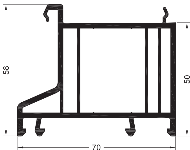
Профиль подставочный 50/70
