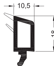
Штапик 10,5
