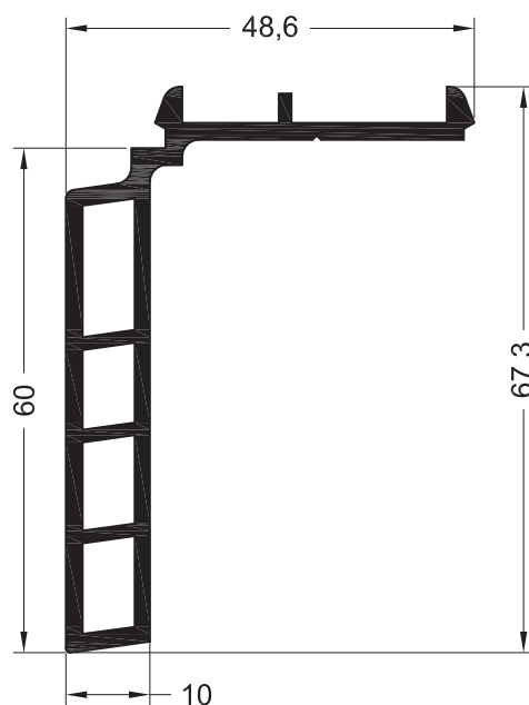
Профиль подставочный 32
