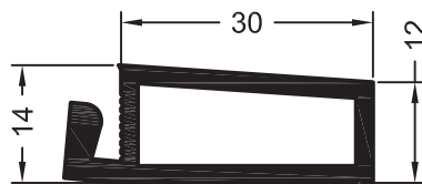
Профиль расширительный
