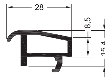
Профиль опорный транспортный
