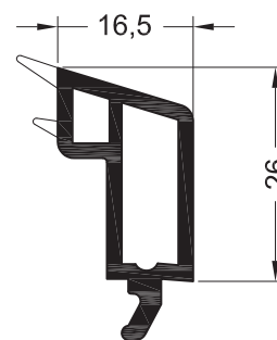
Штапик 16,5 для глухого остекления
