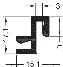
Профиль соединительный
