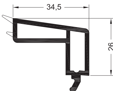
Штапик 34,5 для глухого остекления
