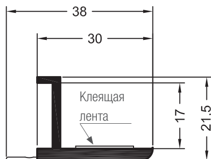
Нащельник 30
