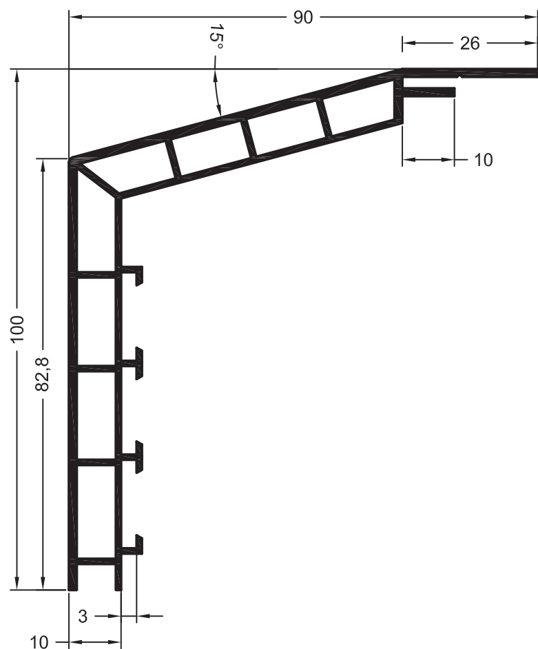
Профиль облицовочный 6
