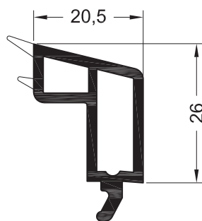
Штапик 20,5 для глухого остекления
