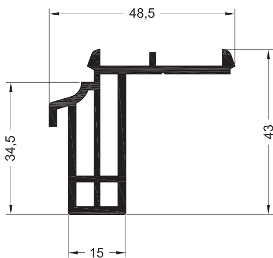
Профиль подставочный 37
