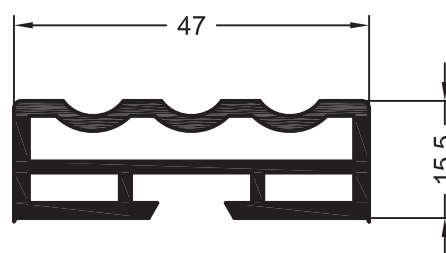
Профиль декоративный 1
