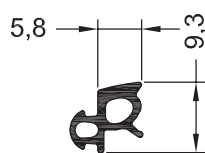
Уплотнение для стекла № 66 1330201 1003 1330201 1004 400 EPDM
