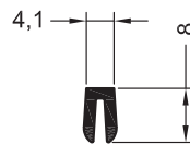
Профиль-заглушка паза штапика 1
