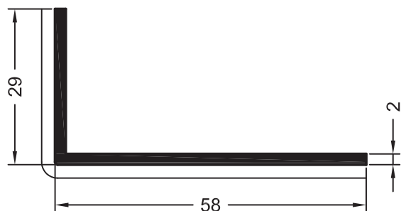
Уголок 1
