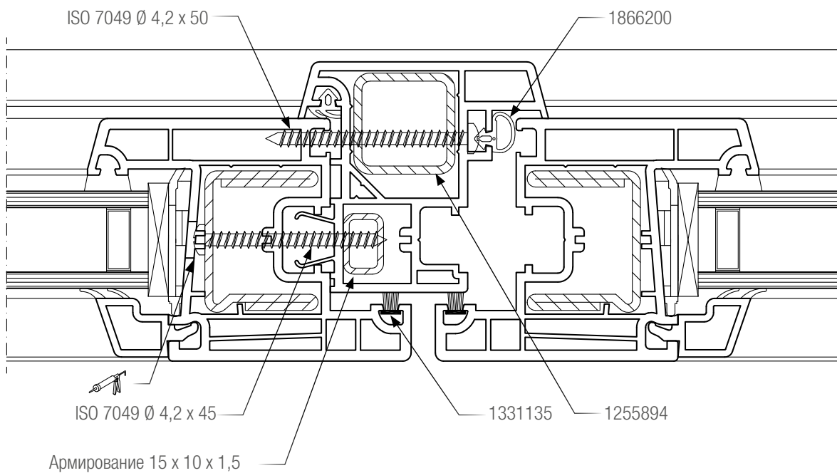
Область стыка двух сдвижных створок, системы 60 мм
