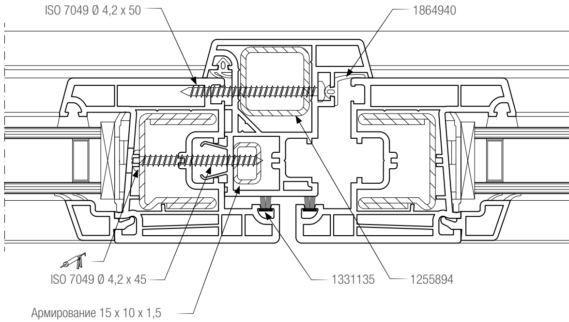
Область стыка поворотной и сдвижной створок, системы 60 мм
