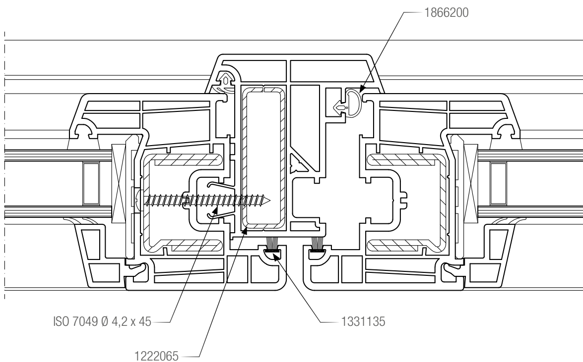
Область стыка двух сдвижных створок, системы 70 мм
